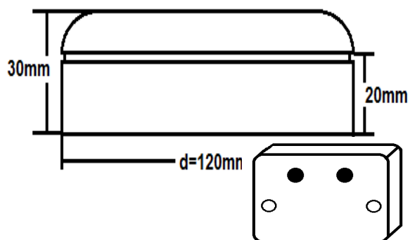
Mit Taster-Dimmer / with touch dimmer
