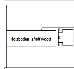
Möbelstück Seitenansicht furniture side view
